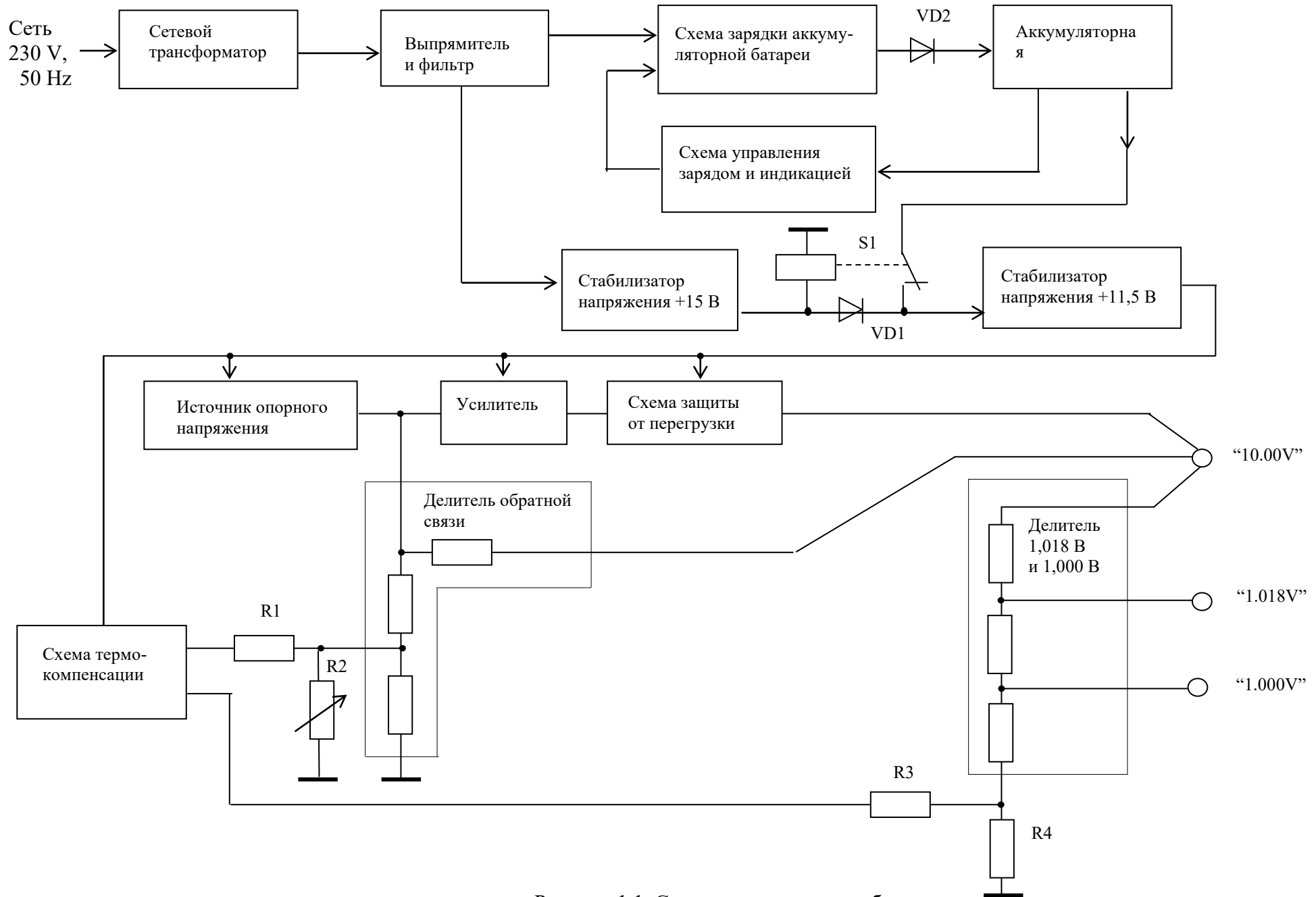
Рисунок 1.1 Структурная схема прибора
