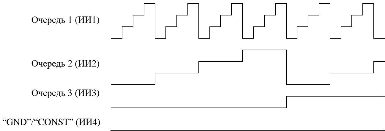
Рисунок 1.6 – Соподчиненная развертка
