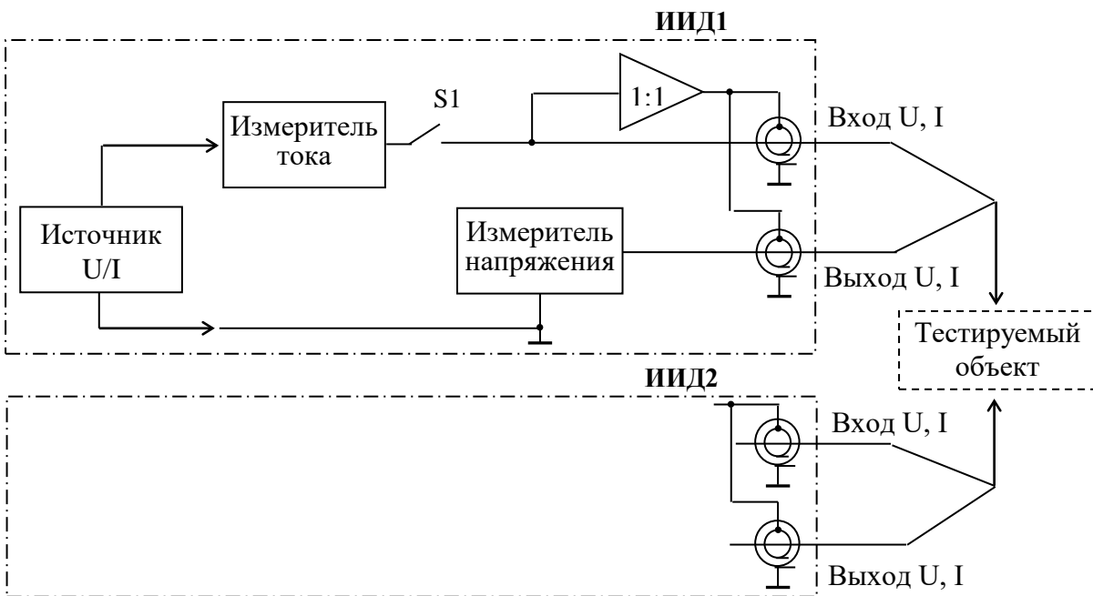
Рисунок 1.3 – Схема структурная ИИО и способ подключения к тестируемому объекту
