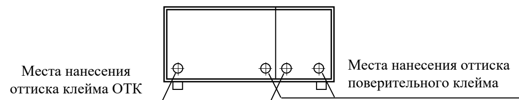
Рисунок 1.18 - Схема пломбирования прибора (вид прибора спереди)
