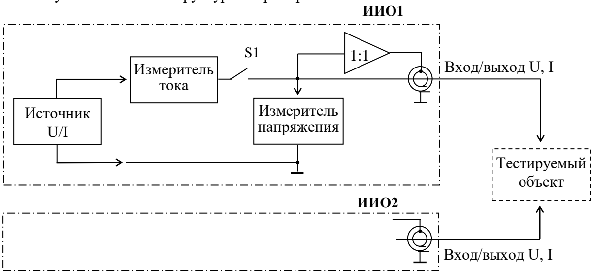
Рисунок 1.2 - Схема структурная прибора
