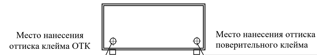
Рисунок 1.19 - Схема пломбирования прибора (вид прибора сзади)
